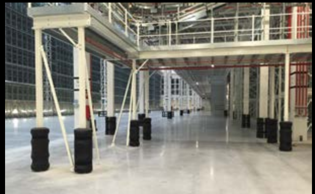
▶ KP 150 / column protection
